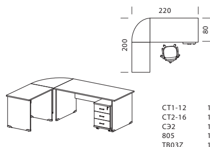
Рабочее место на основе прямоуг. стола 160 x 80
