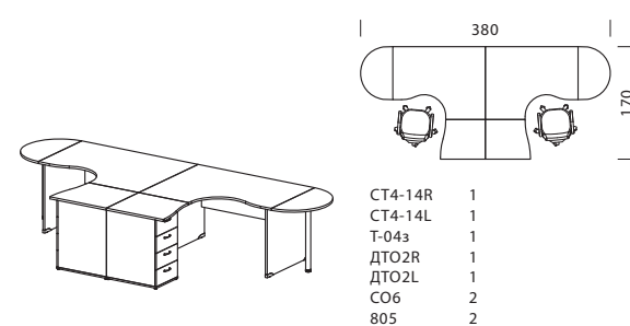
Рабочие места на основе асимметр. стола 140 x 110
