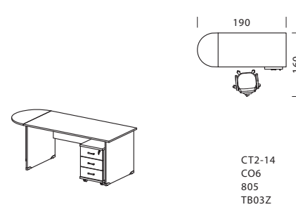
Рабочее место на основе прямоуг. стола 140 x 80
