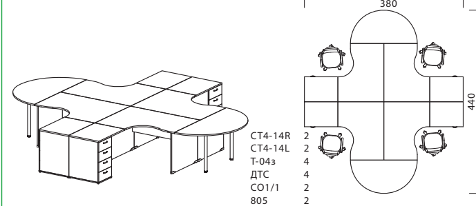
Рабочие места на основе асимметр. стола 140 x 110
