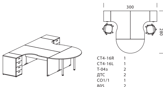
Рабочие места на основе асимметр. стола 160 x 110
