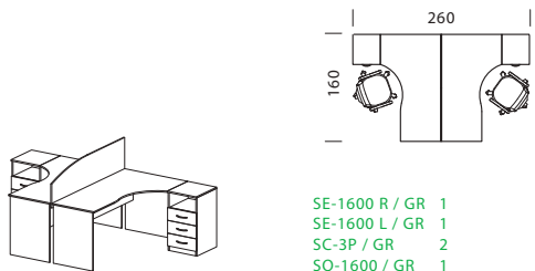
Рабочее место на основе асимметр. столов 160 x 90
