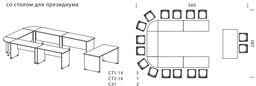
Конференц - стол на 14 мест на основе стола CT1-14 со столом для президиума
