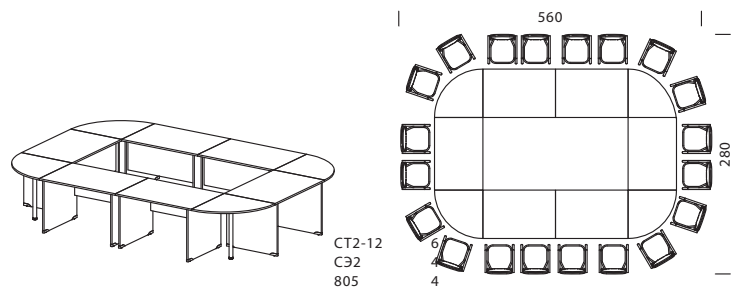
Конференц - стол на 20 мест на основе стола СТ2-12
