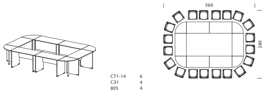
Конференц - стол на 14 мест на основе стола CT1-14
