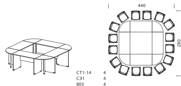
Конференц - стол на 16 мест на основе стола CT1-14
