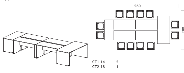
Конференц - стол на 10 мест и стол руководителя на основе стола СТ1-14
