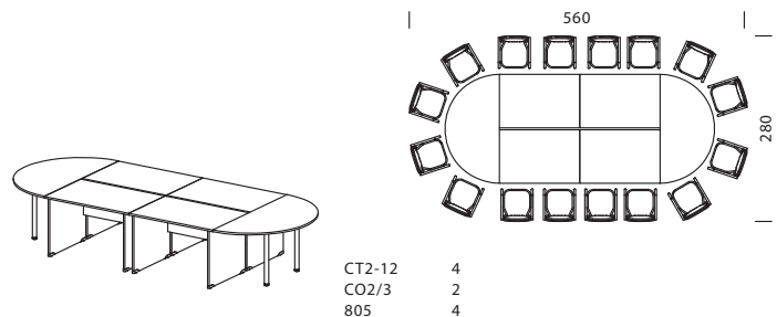
Конференц - стол на 16 мест на основе стола CT2-12
