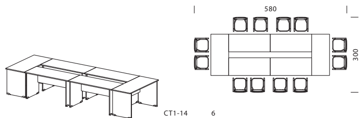
Конференц - стол на 12 мест на основе стола СТ1-14
