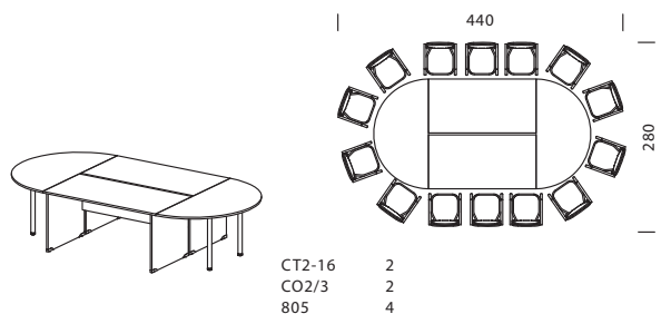
Конференц - стол на 14 мест на основе стола CT2-16
