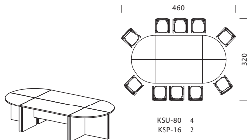
Конференц - стол на 8-10 мест
