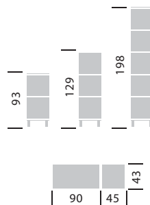
Рис.1 . Высота, ширина и глубина модулей
