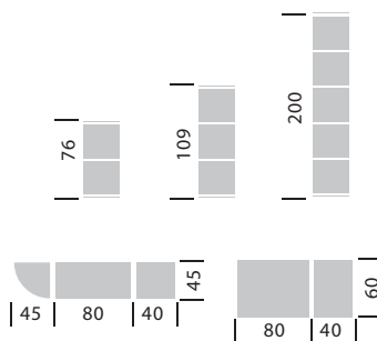
Рис.1 . Высота, ширина и глубина модулей
