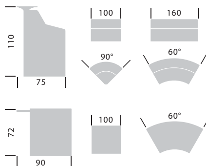
Рис.1 . Высота, ширина и глубина модулей
