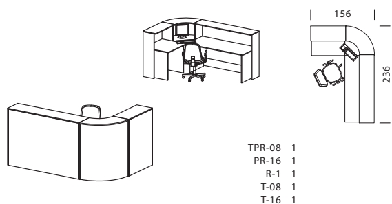
Стойка для зоны приветствия угловая на 1 рабочее место
