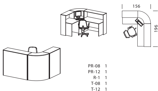
Стойка для зоны приветствия угловая на 1 рабочее место
