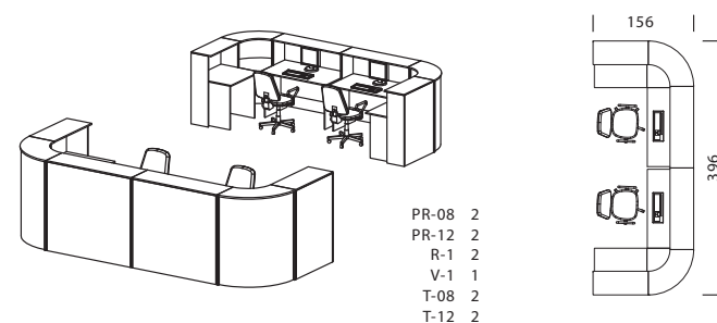
Стойка для зоны приветствия U-образной конфигурации на 2 рабочих места
