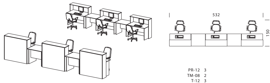
Стойка для зоны приветствия типа "линия" с перепадом высоты на 3 рабочих места
