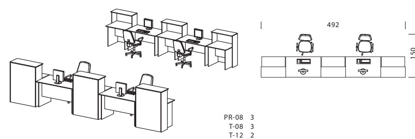
Стойка для зоны приветствия типа "линия" с перепадом высоты на 2 рабочих места
