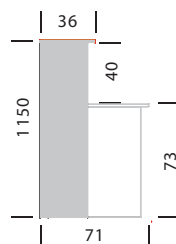
Рис.2 Основные размеры стоек
