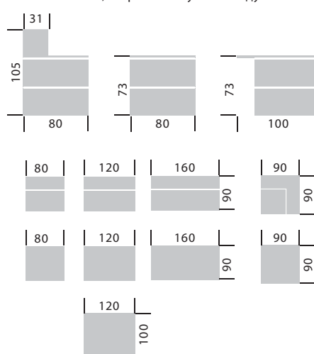
Рис.1 . Высота, ширина и глубина модулей
