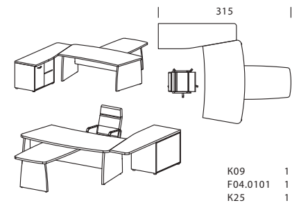
Рабочее место на основе стола 199 x 100 см на панельном каркасе
