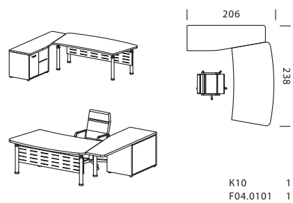
Рабочее место на основе стола 199 x 100 см на металлических опорах
