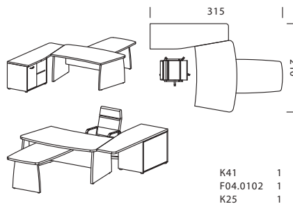
Рабочее место на основе стола 170 x 100 см на панельном каркасе
