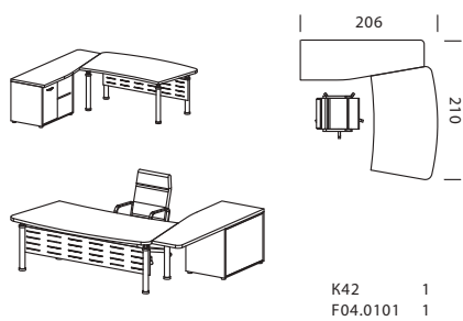
Рабочее место на основе стола 170 x 100 см на металлических опорах
