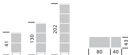
Рис.2 . Высота, ширина и глубина модулей
